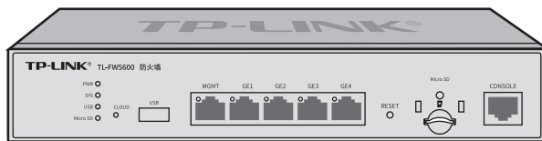
图1-3 TL-FW5600前面板示意图
